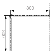
Barra de apoio em "L" piso 80x80 1 1/4" 23010 - Cód.: 7006
