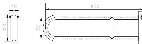
Barra de apoio lateral articulada 80cm 1 1/4 23025- Cód.: 7013
