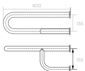
Barra apoio lateral parede com fixação lado direito 80cm 1 1/4" 23021 - Cód.: 7010
