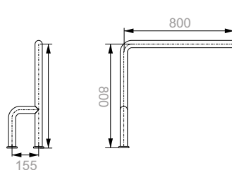
Barra de apoio em "L" piso lado esquerdo 80x80 1 1/4" 23012 - Cód.: 7008
