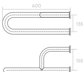
Barra apoio lateral parede com fixação lado esquerdo 60cm 1 1/4" 23022 - Cód.: 7011
