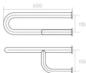
Barra apoio lateral parede com fixação lado direito 60cm 1 1/4" 23020 - Cód.: 7009
