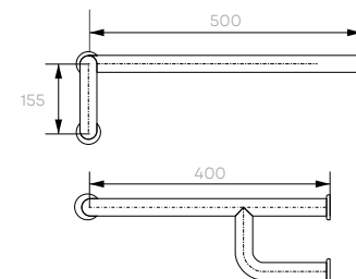
Barra de apoio em "L" parede lado esquerdo 50x40cm 1 1/4" 23033 - Cód.: 7005
