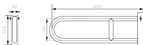
Barra de apoio lateral articulada 60cm 1 1/4 23024- Cód.: 7003
