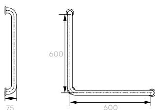
Barra de apoio em "L" parede 60x60cm 1 1/4" 23060 - Cód.: 4714
